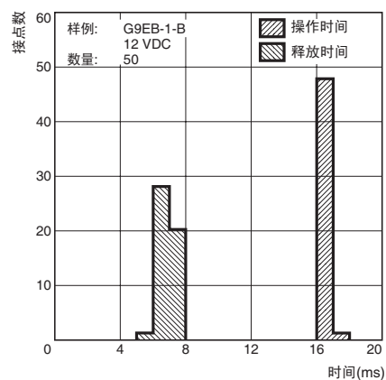
时间特性分布
