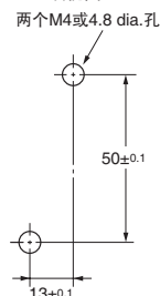
安装孔尺寸 (顶视图)
