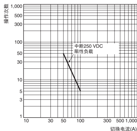
电气寿命（中断性能）
