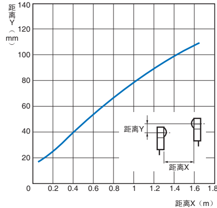
平行移动特性
