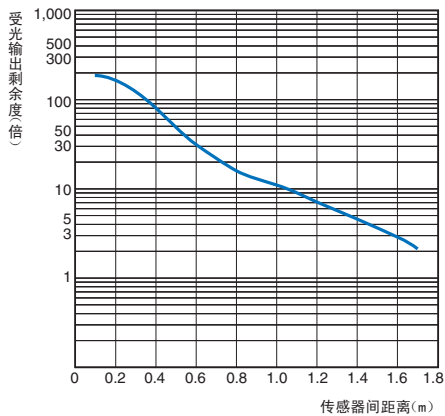
受光输出剩余度—距离特性
