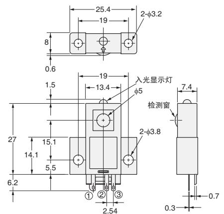
端子配置
