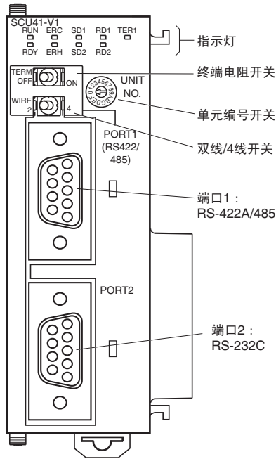
CJ1W-SCU41-V1
