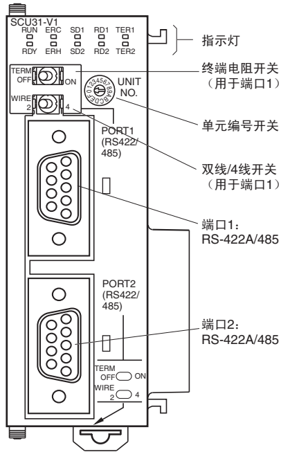
CJ1W-SCU31-V1
