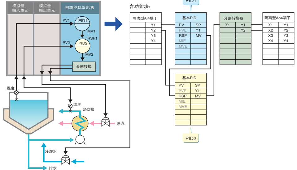
● 示例：串级控制（加热/冷却）
