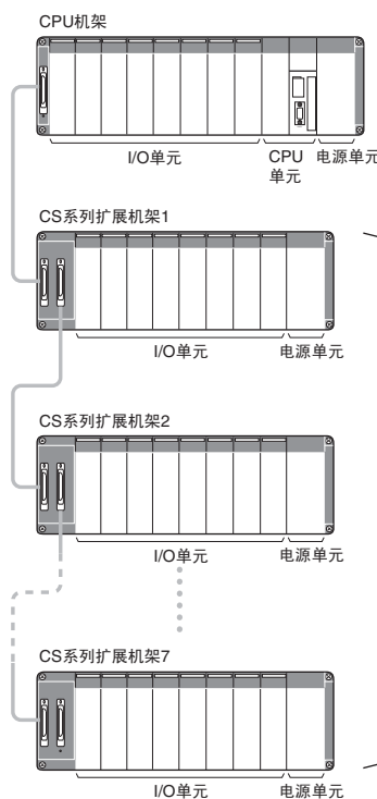
可以最多连接七个扩展机架。
