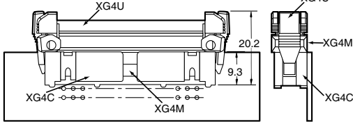
XG4U+XG4M+XG4C（L形端子）
