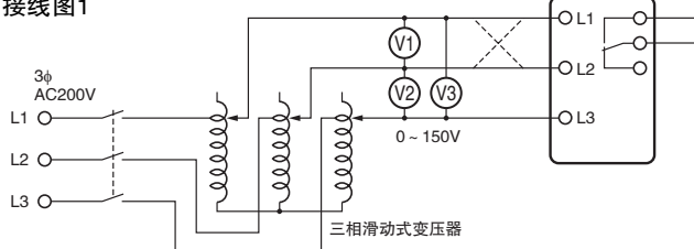
接线图1
