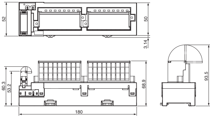
安装DCN4-TB4开放型连接器时
