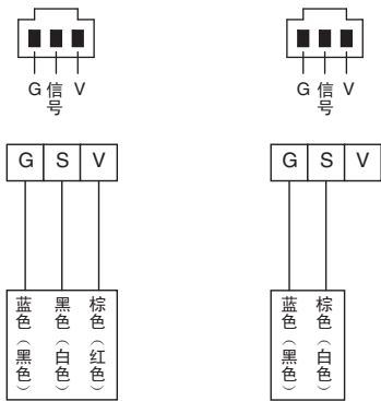
3线传感器，带NPN输出 (光电传感器或接近传感器)
