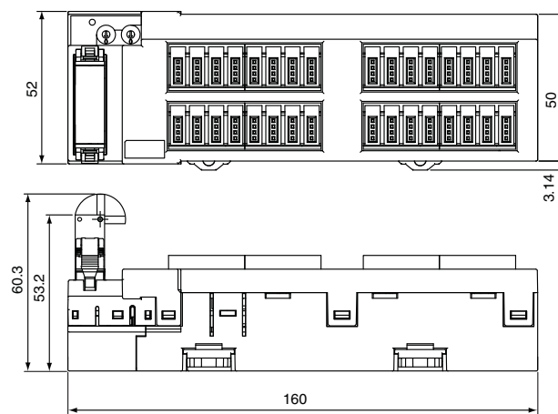
安装DCN4-TB4开放型连接器时
