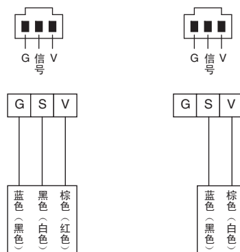
3线传感器，带PNP输出 (光电传感器或接近传感器)
