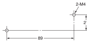
安装孔加工尺寸图
