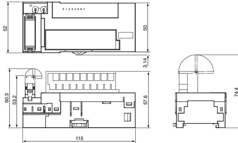
安装DCN4-TB4开放型连接器时
