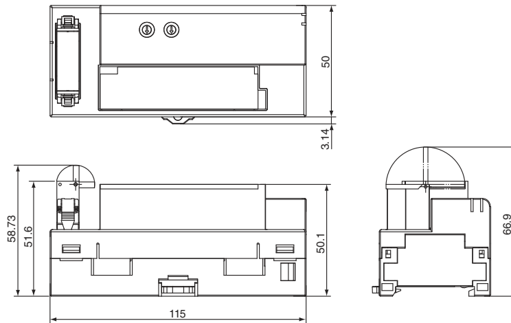
安装DCN4-TB4开放型连接器时
