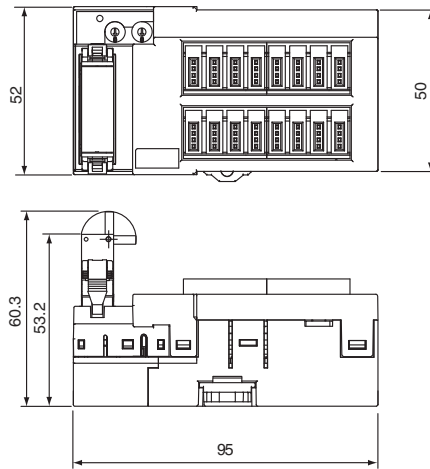
安装DCN4-TB4开放型连接器时
