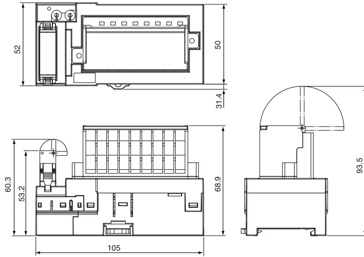
安装DCN4-TB4开放型连接器时
