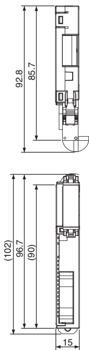
安装DCN4-TB4开放型连接器时
