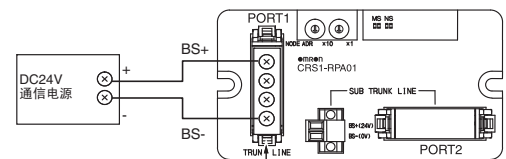
此处连接开放型连接器。
