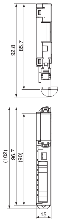
安装DCN4-TB4开放型连接器时
