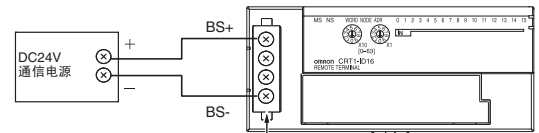
此处连接开放型连接器。
